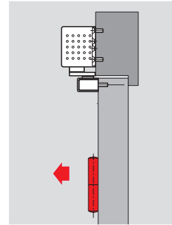
Kozijndorpelmontage scharnierzijde
